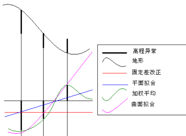
图 4-13 高程拟合平面模拟对比图
