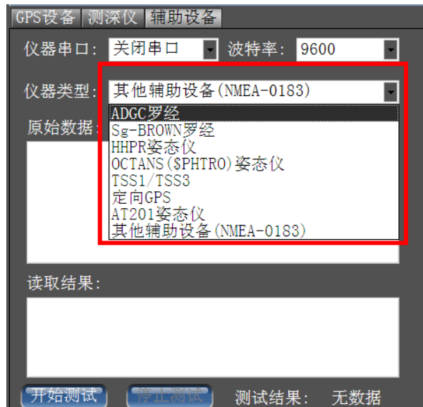
图 5-13 辅助传感器仪器类型
