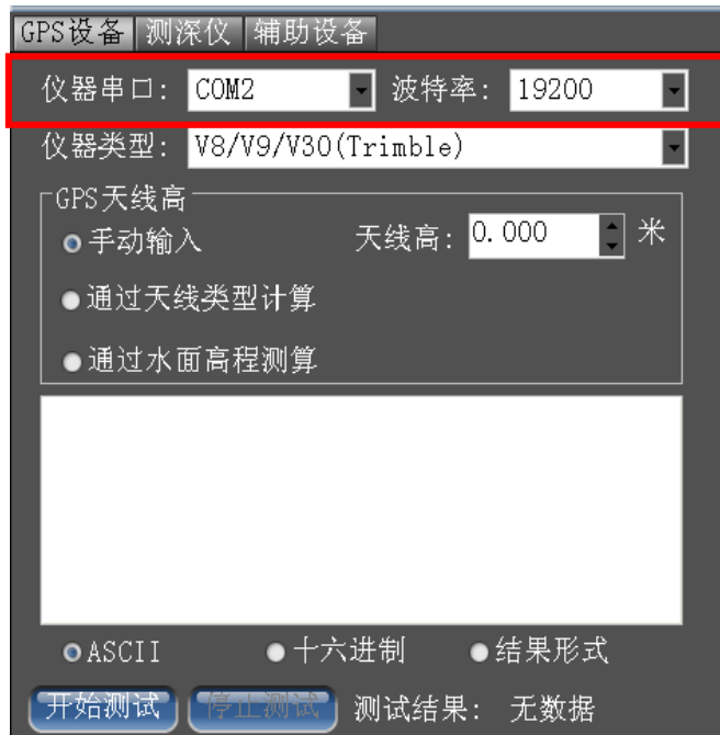
图 5-1 GPS 串口设置
